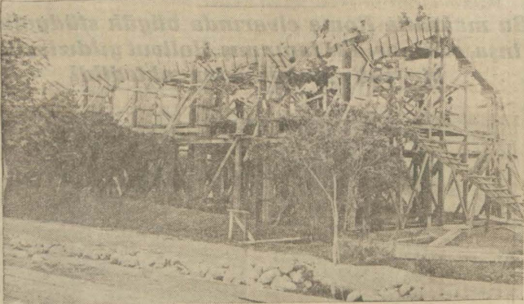
Malatyada inşaat başlanılan mensucat fabrikasının inşaatı bir hayli ilerlemiştir. Resimde fabrikanın beton sütunlarının döküleceği kalıpların hazırlanmış olduğu görülmektedir.
